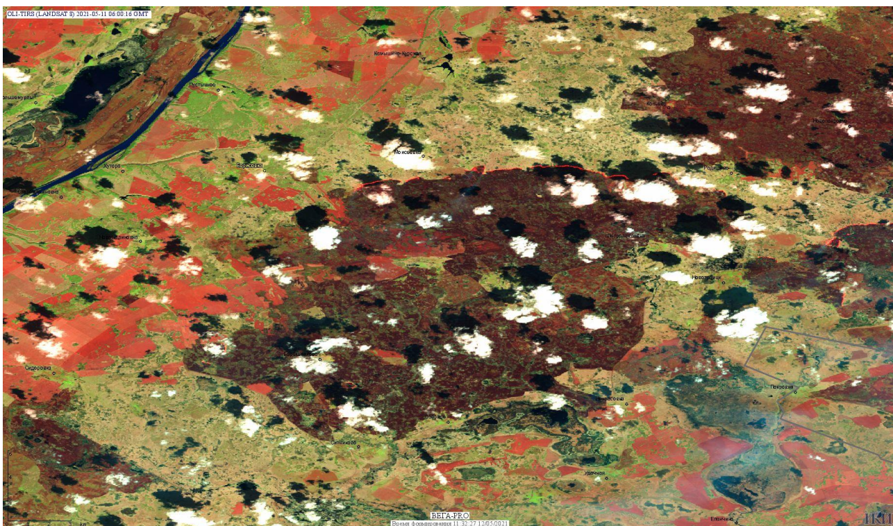
Рис. 3 Пожары и сельскохозяйственные палы в Нижнеомском районе Омской области. Данные Landsat 8.
