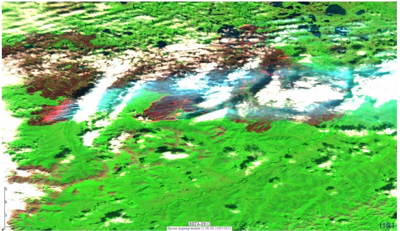
Рис. 4 Пожары в Пенжинском районе Камчатского края. Данные Landsat 8
