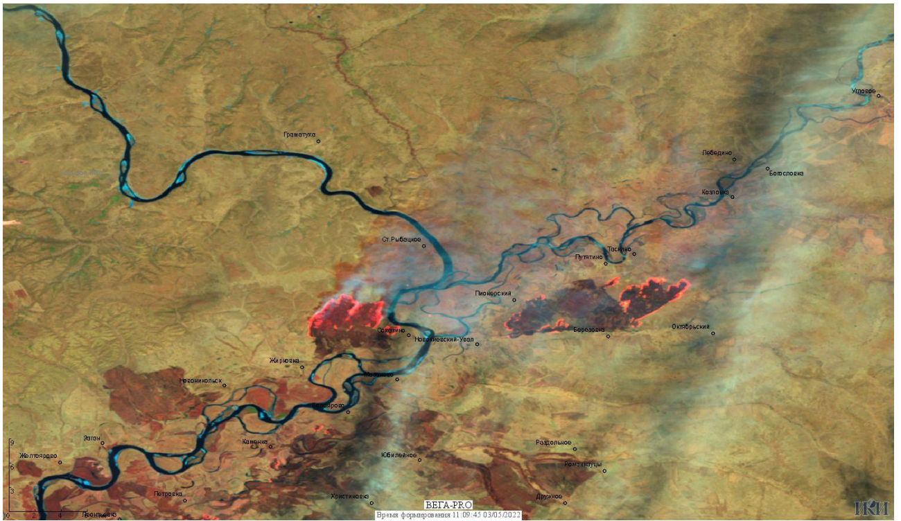
Рис. 4 Пожары и сельскохозяйственные палы в Мазановском районе Амурской области. Данные Landsat 8.
