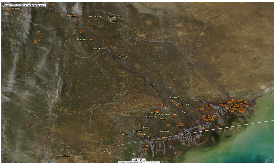
Рис. 1 Пожары и сельскохозяйственные палы в Астраханской области
